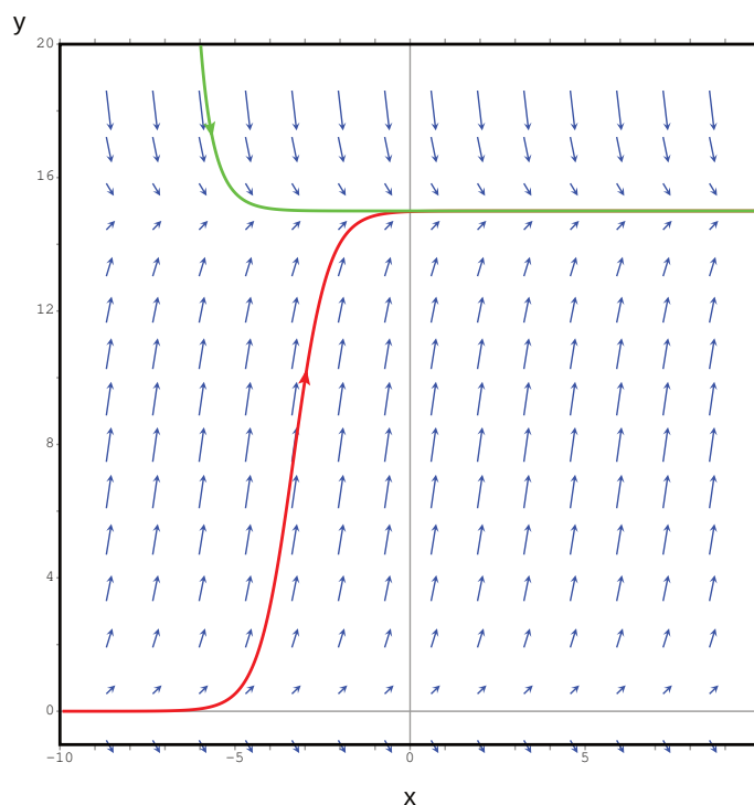
FIGURE XVIII2 – Graphe réalisé avec le logiciel Maxima
