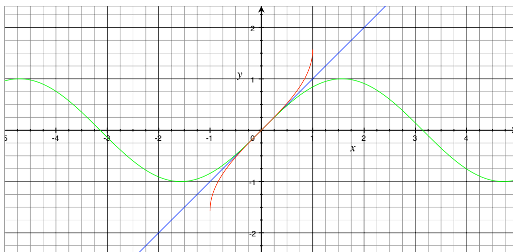
FIGURE IX4 – Graphes de sin et arcsin
