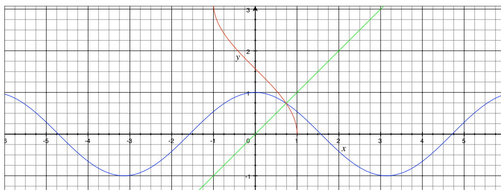
FIGURE IX5 – Graphes de cos et arccos
