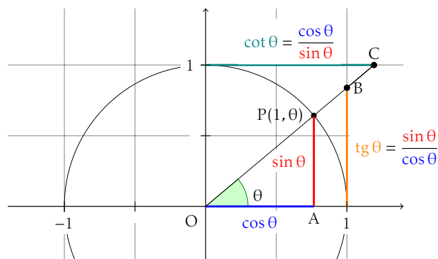
FIGURE VI3 – Illustration des fonctions sinus, cosinus, tangente et cotangente sur le cercle trigonométrique (ici, pour l'angle \theta = 2\pi/9 soit 40^\circ ).
