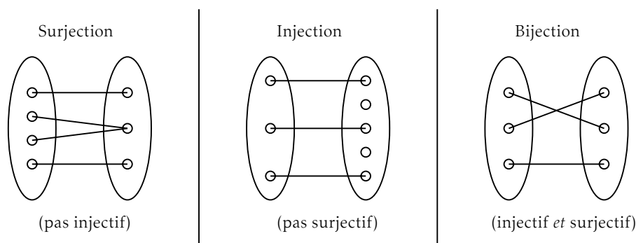
FIGURE IV3 – Injectivité, surjectivité.
