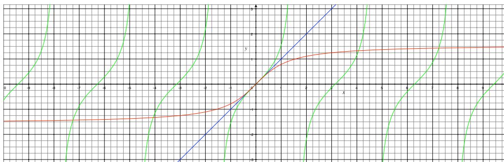
FIGURE IX6 – Graphes de tg et arctg
