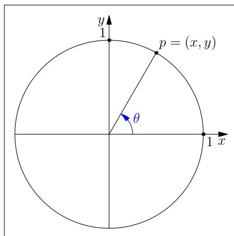
FIGURE IX3 – Le cercle trigonométrique
